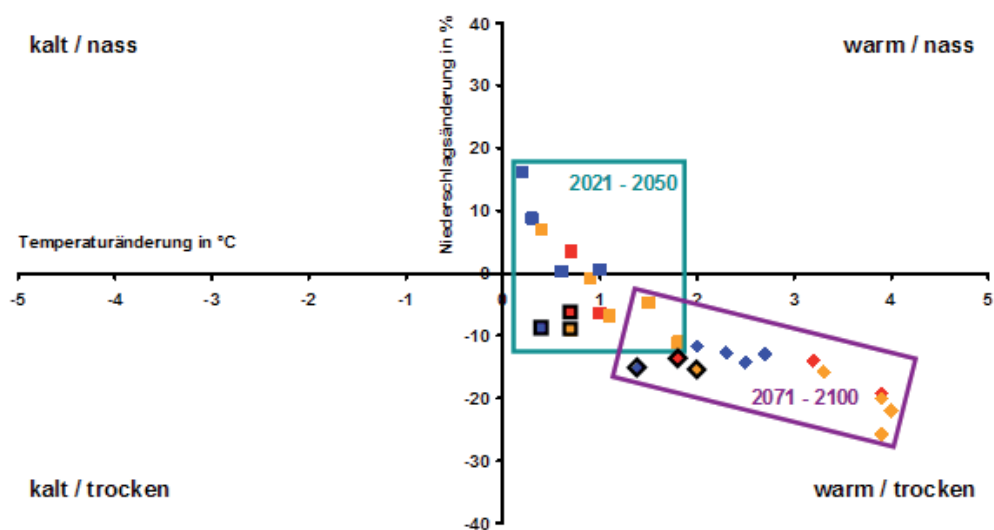
Abbildung 6: Tagesmitteltemperatur - Beispiel einer Klimaprojektion
