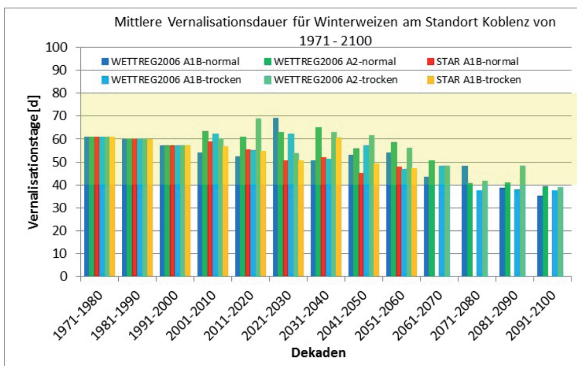
Abbildung 21: Mittlere Vernalisationsdauer für Winterweizen
