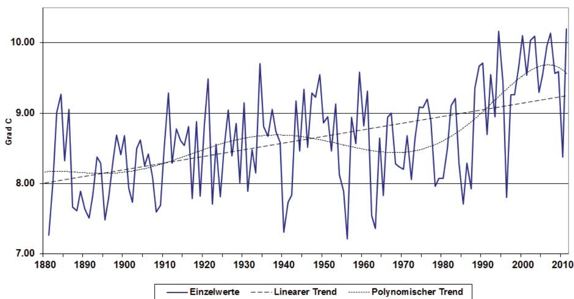
Abbildung 3: Beobachtete Jahresmitteltemperaturen in Rheinland-Pfalz ab 1881
