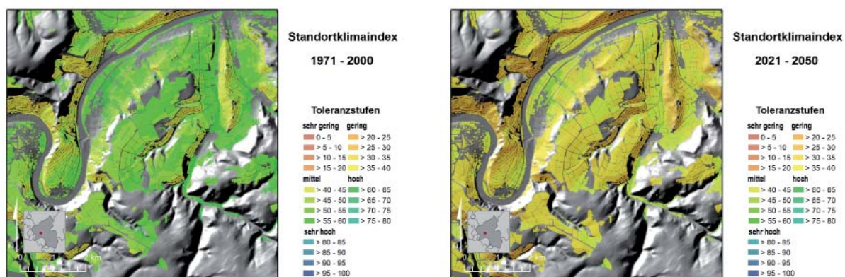
Abbildung 19: Standortklimaindex auf landwirtschaftlich genutzten Standorten an der Mittelmusel
