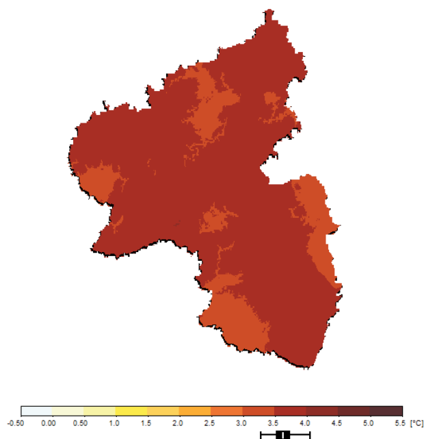
Abbildung 7: Thermopluviogramm - Abweichung von Jahrestemperatur und Niederschlag im Sommer
