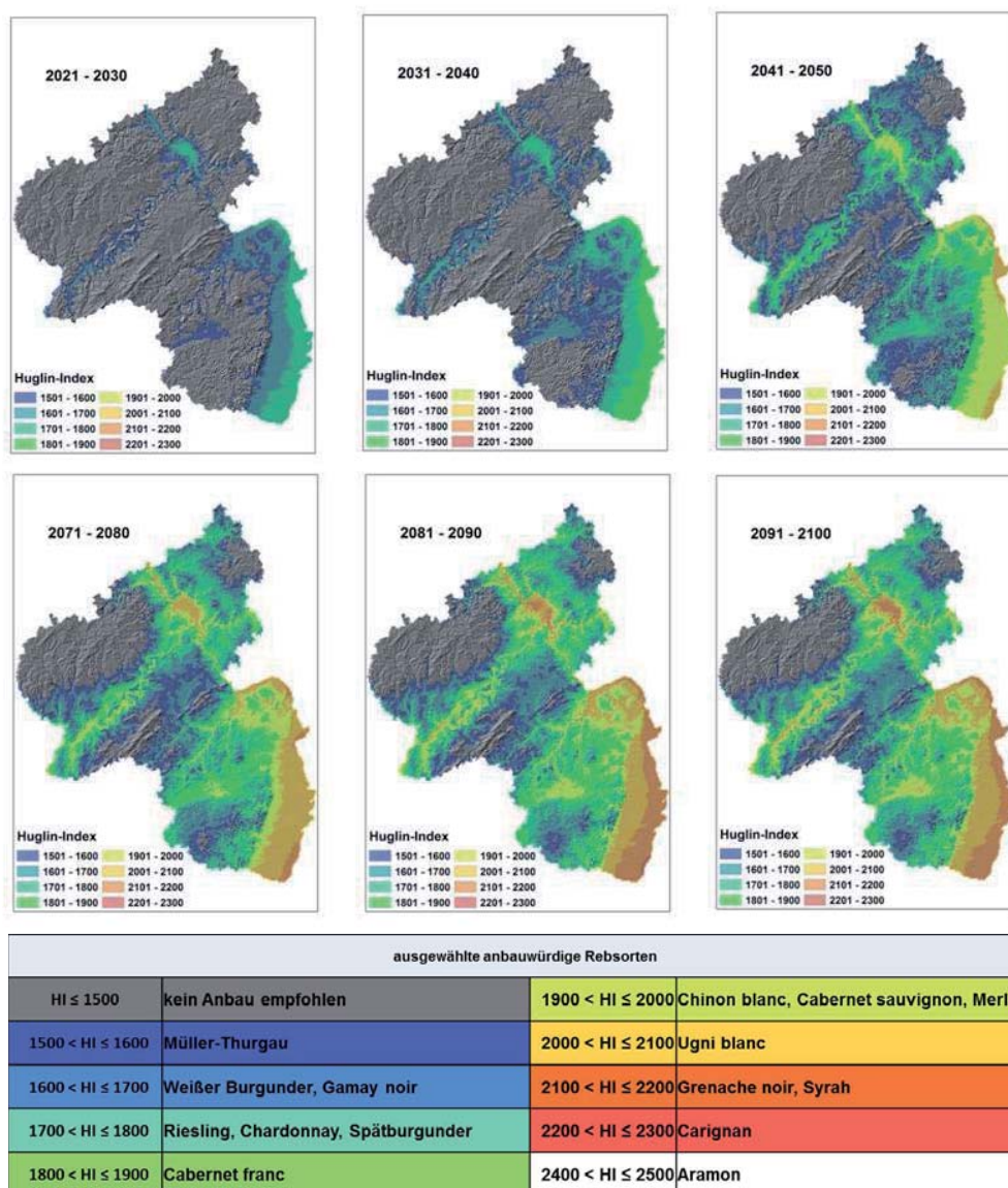
Abbildung 24: Zeitschnitte für die zukünftige Entwicklung des Huglin-Index in Rheinland-Pfalz (Projektion: WETTREG2006 A1B-trocken)
